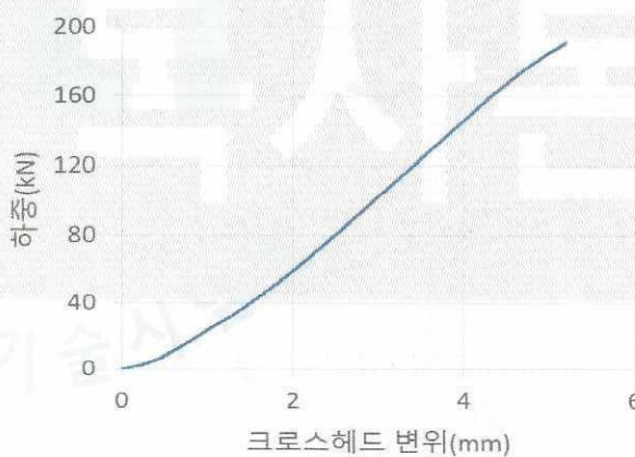
그림 3. 시험 그래프
